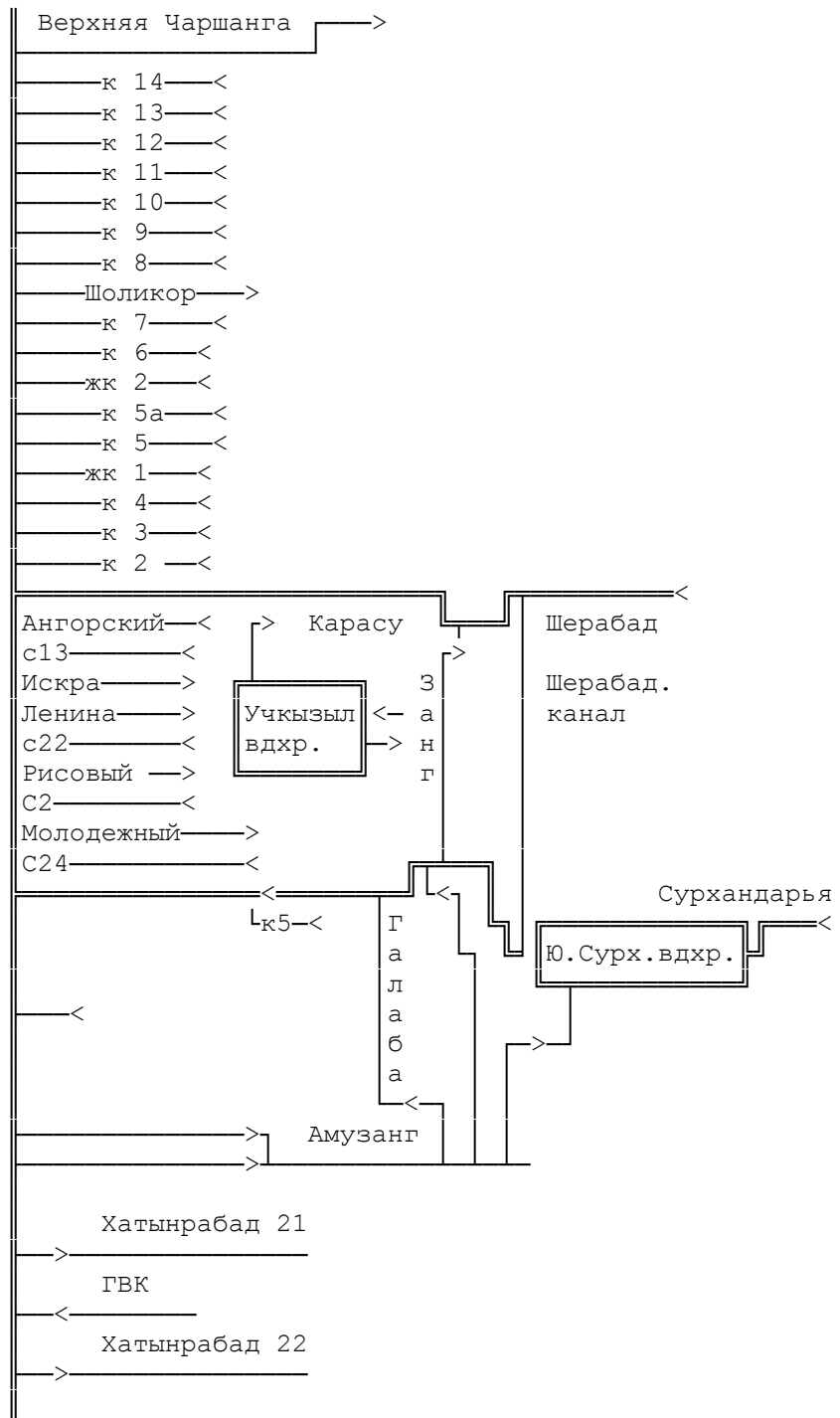
РИС Л И Н Е Й Н А Я С Х Е М А А М У Д А Р Ь И ( Ч Е Т В Е Р Т А Я Ч А С Т Ь )
